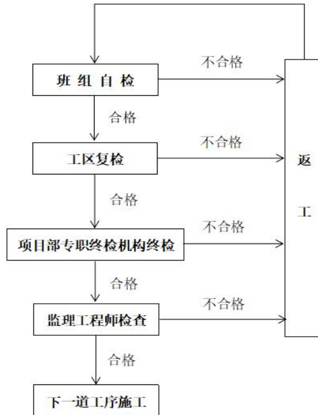
质检程序图
